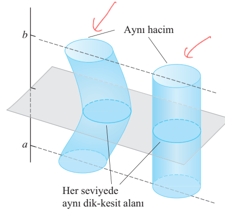
ŞEKİL 6.6 Cavalieri Prensipli: Bu katı cisimlerin hacimleri aynıdır. Bunu bozuk paralarla kendi kendinize görebilirsiniz (Örnek 2).
