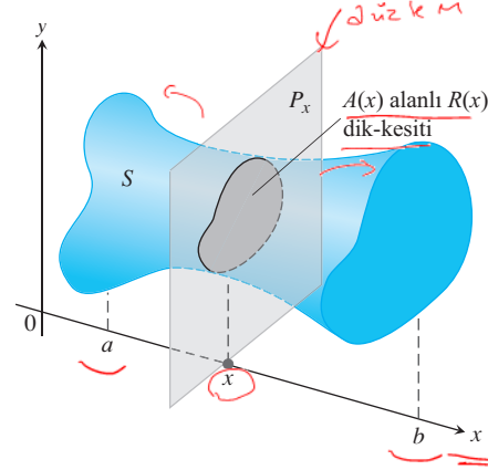
ŞEKİL 6.1 S katı cisminin, [a, b] aralığındaki bir x noktasında x -eksenine dik olan bir P_x düzlemi ve S 'nin kesişimiyle oluşan dik-kesiti.
